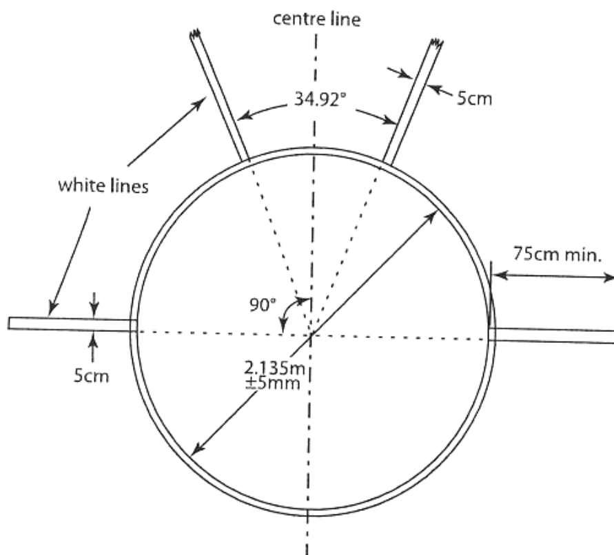
Mynd 14 - Sleggjuhringur
