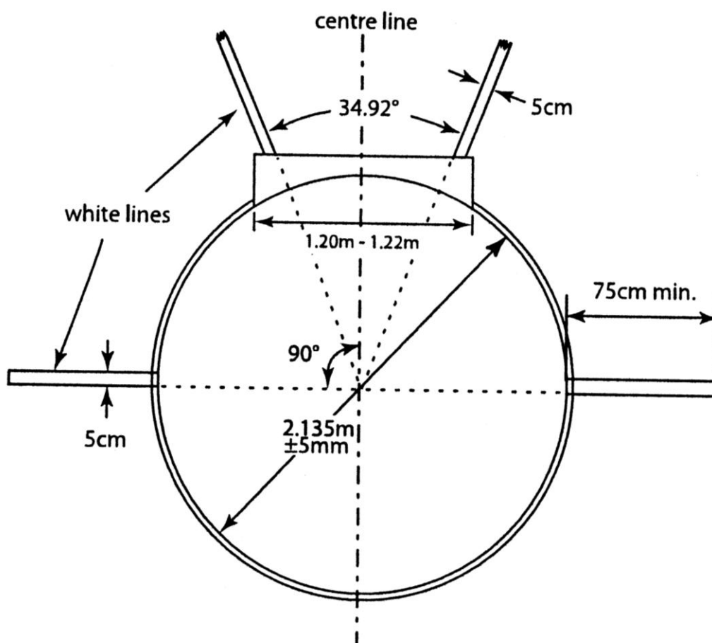
Mynd 12 - Kúluvarpshringur
