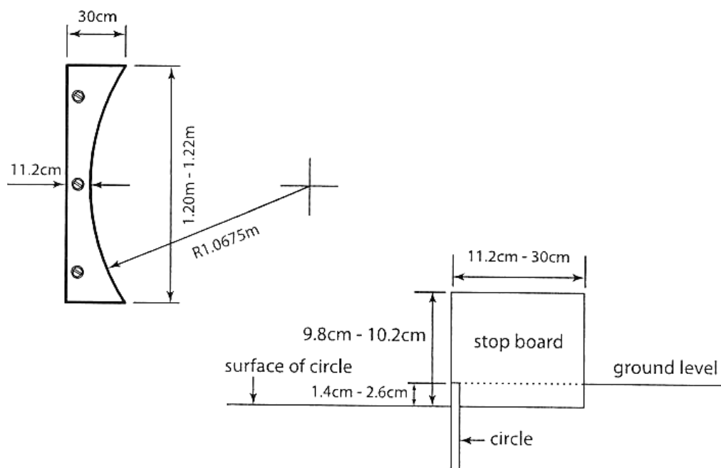
Mynd 17 – Stilliplanki
