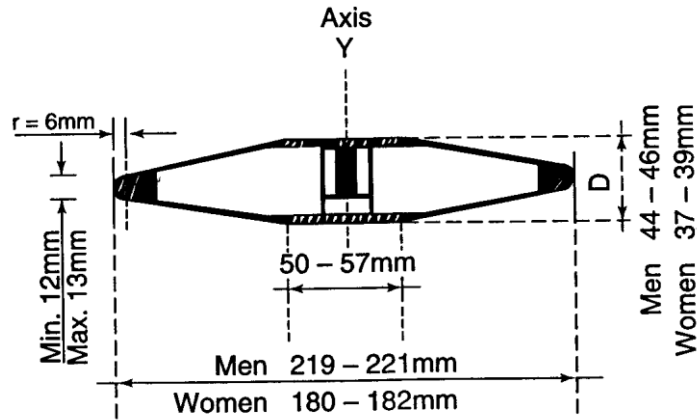
Mynd 18 – Kringla
