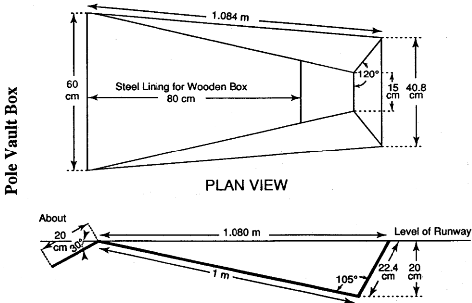
Mynd 7 – Stangarstökkstokkur
