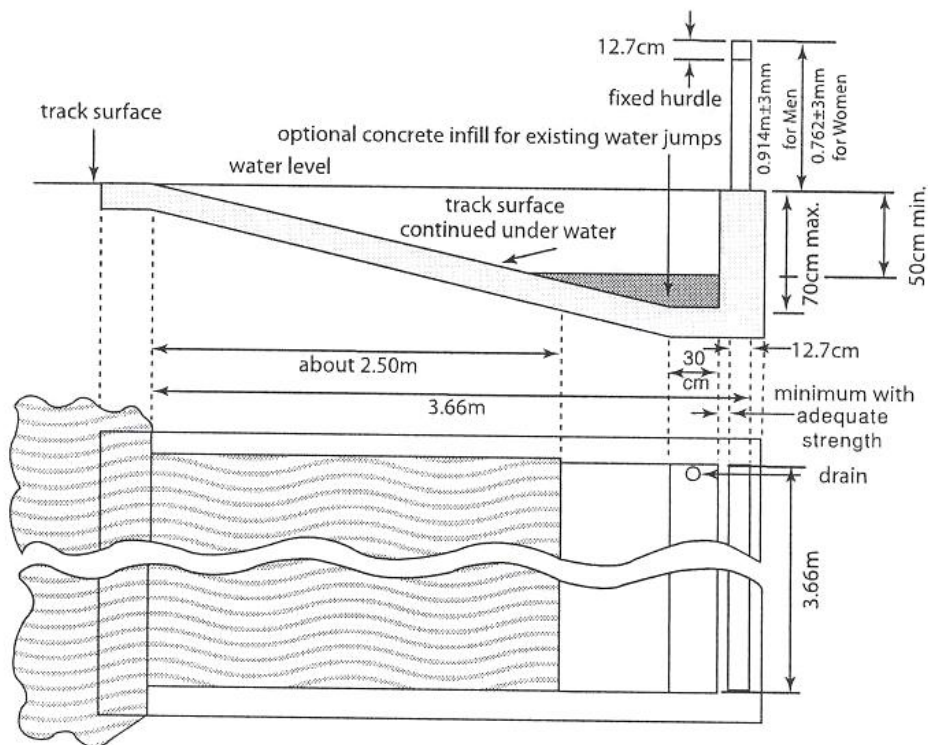
Mynd 4 - Vatnsgrýfja
